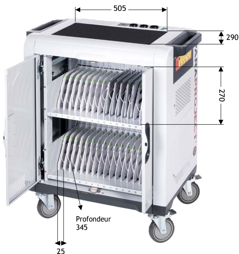
Dimensions en mm
